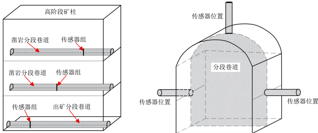
图4 微震传感器组布置示意图
