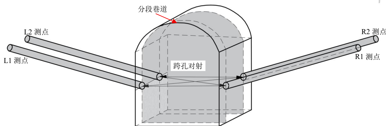
图5 超声波层析成像监测孔布置示意图
