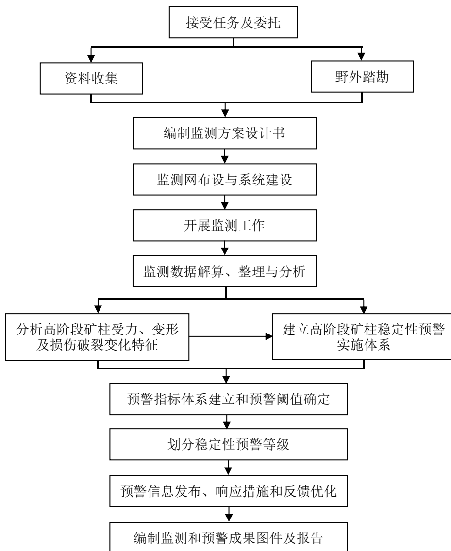
图 1 监测与预警实施流程图
