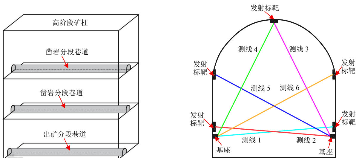
图2 高阶段矿柱内部凿岩和出矿分段巷道位置和断面收敛位移监测点布置示意图
