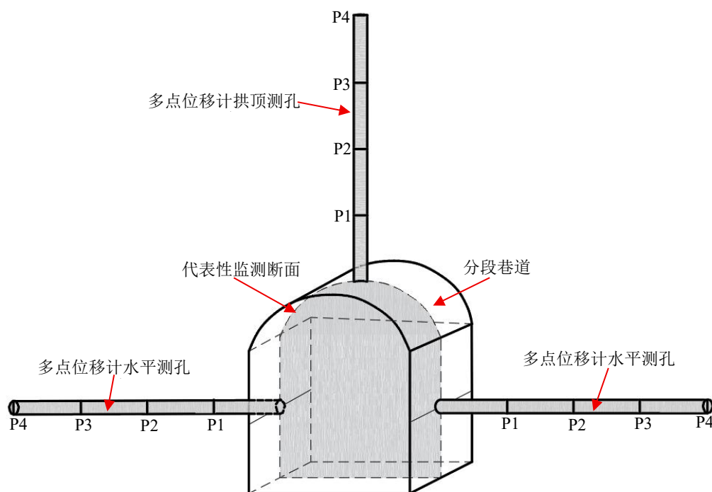
图3 多点位移计测点布置示意图
