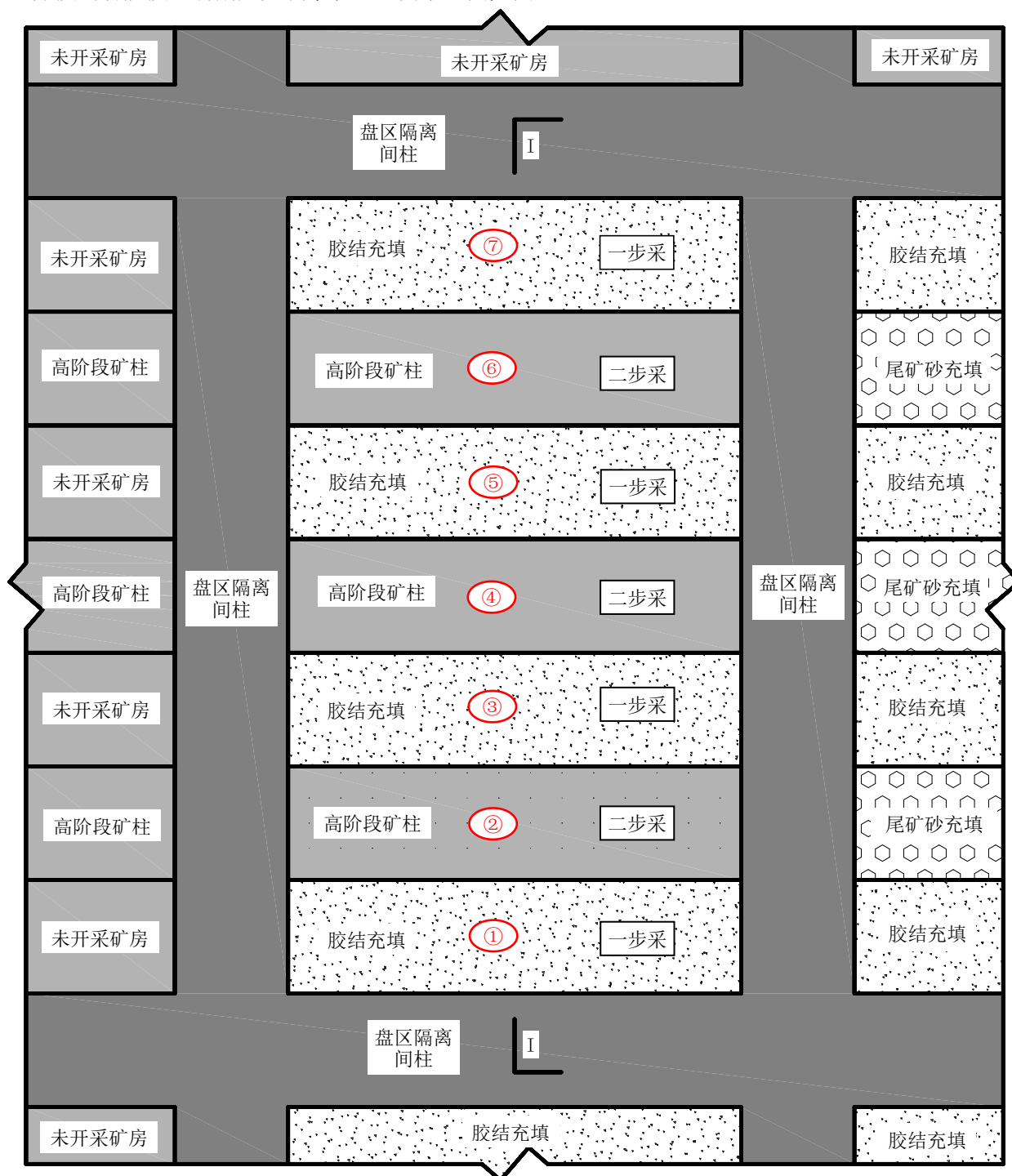
图A.1 分段凿岩阶段空场嗣后充填采矿法平面示意图
