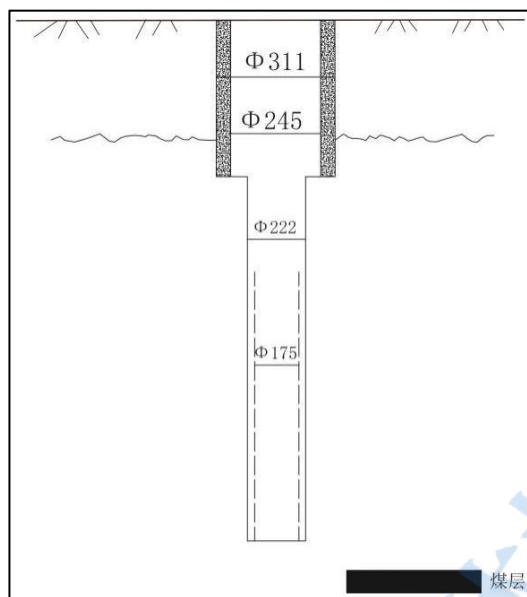
图A. 1 地面直通式导流孔孔径结构图 (mm)
