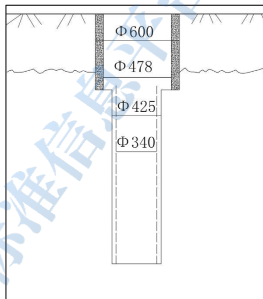
图A. 2 地面抽排钻孔孔径结构图 (mm)
