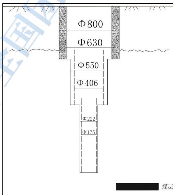
图 A. 3 地面抽泄钻孔孔径结构图 (mm)
